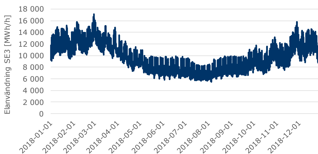
Figur 11. Elanvändningen per timme i SE3 under 2018 (Källa: Svk/Nord Pool)
